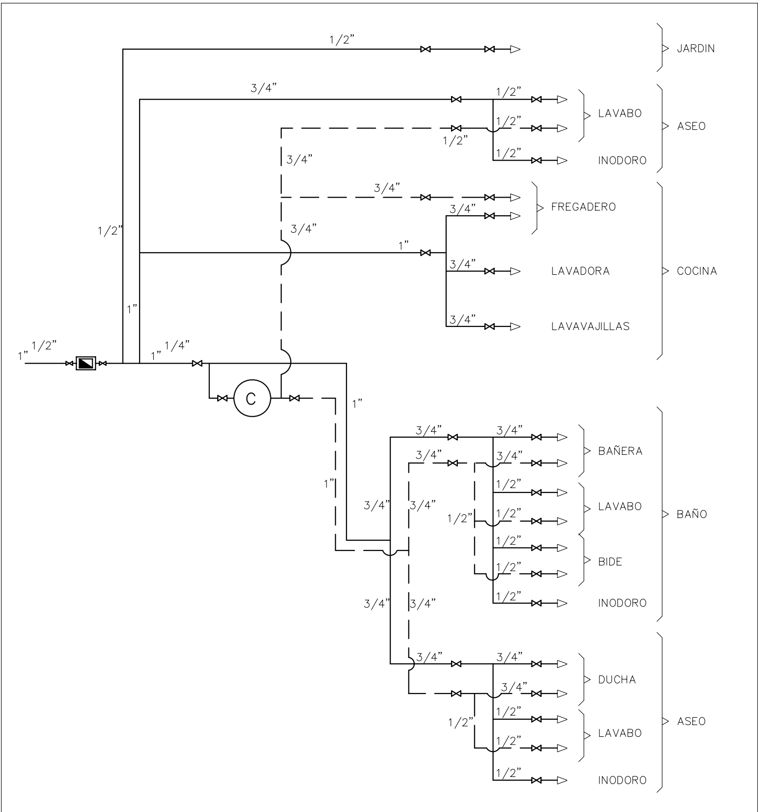
ESQUEMA FONTANERIA INTERIOR
