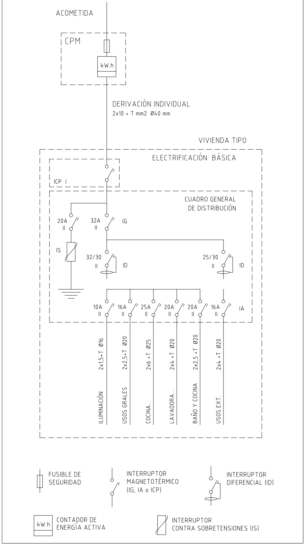
ESQUEMA GENERAL UNIFILAR DE VIVIENDA UNIFAMILIAR
